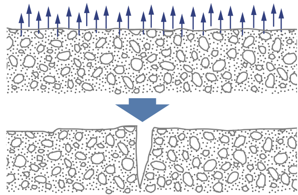
Schrumpfen des plastischen Betons kann durch den Unterdruck, der beim Austrocknen in den mit Flüssigkeit gefüllten Poren entsteht, zu Rissen führen.
