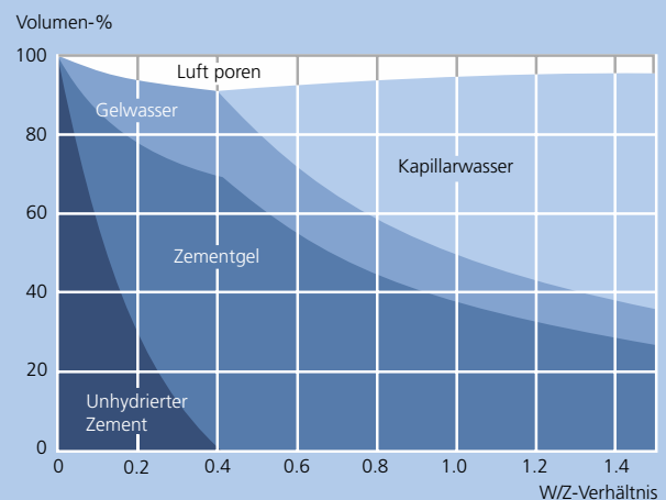
Die Volumenverhältnisse für hydratisierten Zementleim
